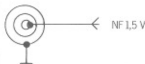
Abb. 5: Beschaltung der NF-Ausgangsbuchse in Schalterstellung „1,5 V“.
